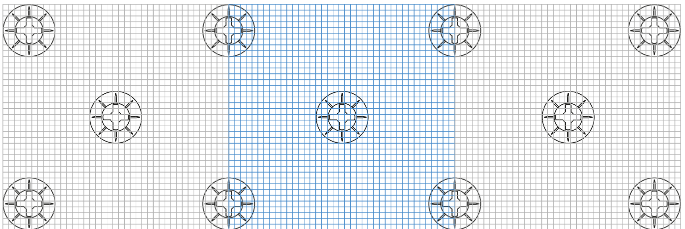
Eksempel på placering af Flexi Level under gangbro ( Illustreret med 3 riste )
